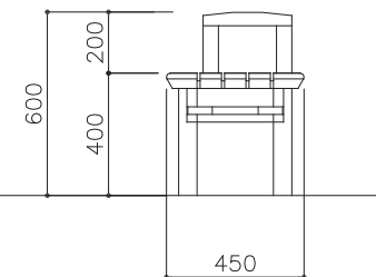
■ 側 面 図
