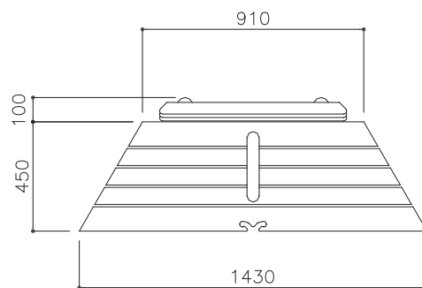
■ 正 面 図
