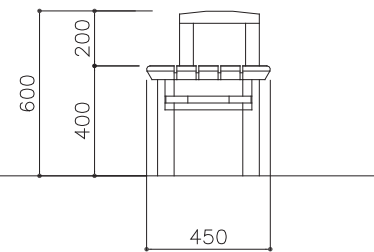
■側面図
